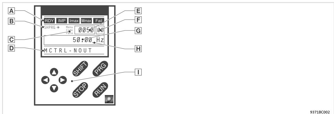
Fig.3-2 Elementi del display e tasti funzione della Tastiera XT EMZ9371BC
