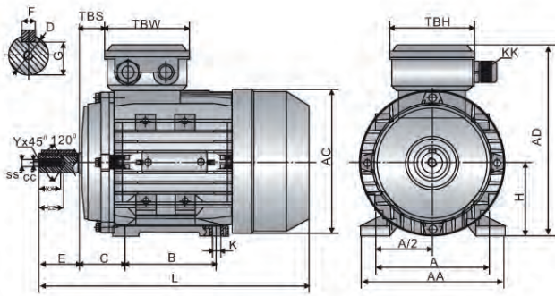
Montaggio B3
