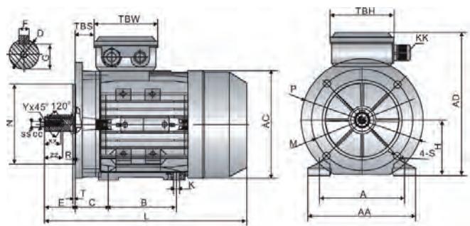
Montaggio B35
