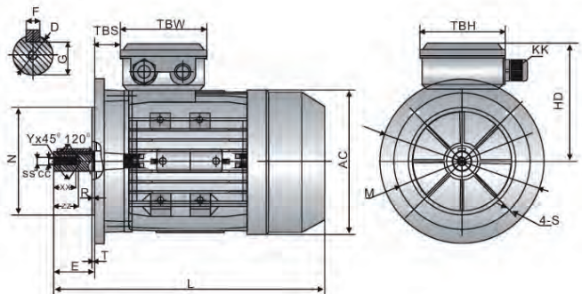
Montaggio B5
