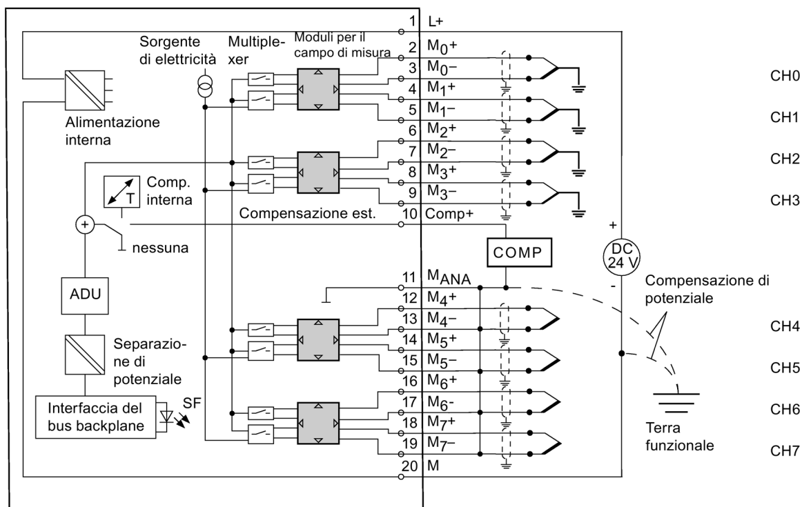
Figura 6-16 Schema di principio e di collegamento
