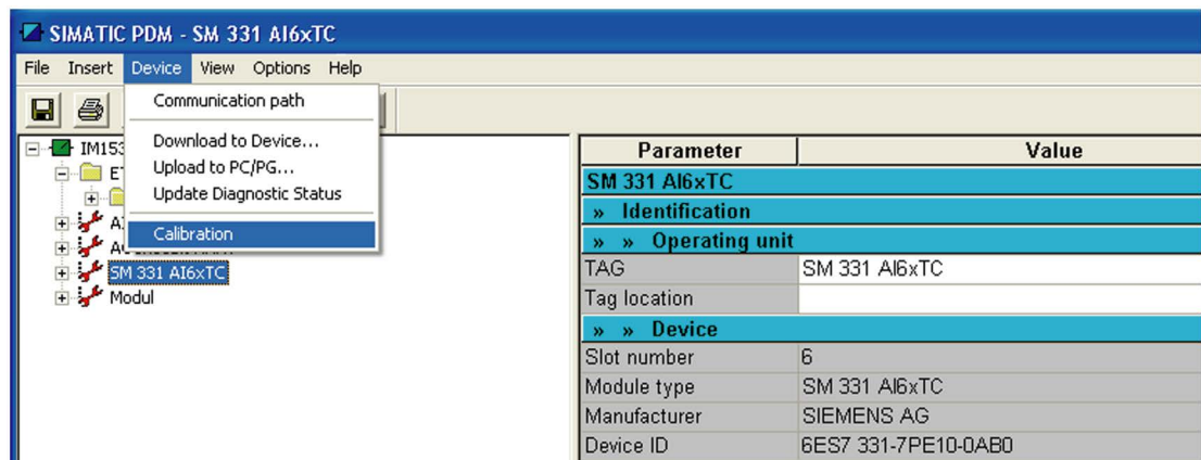
Figura 6-37 Funzione di calibrazione
