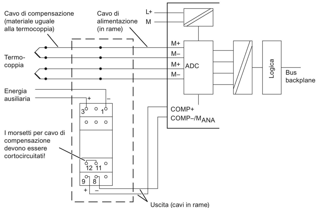
Figura 4-16 Collegamento di termocoppie al giunto freddo
