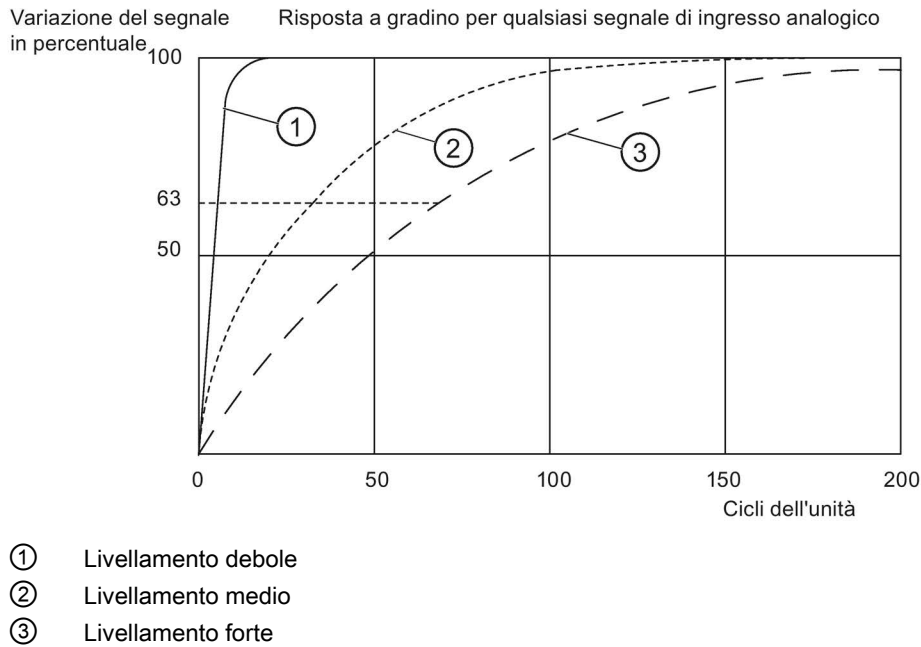
Figura 5-6 Esempio dell'influenza del livellamento sulla risposta a gradino di AI 6 x TC
