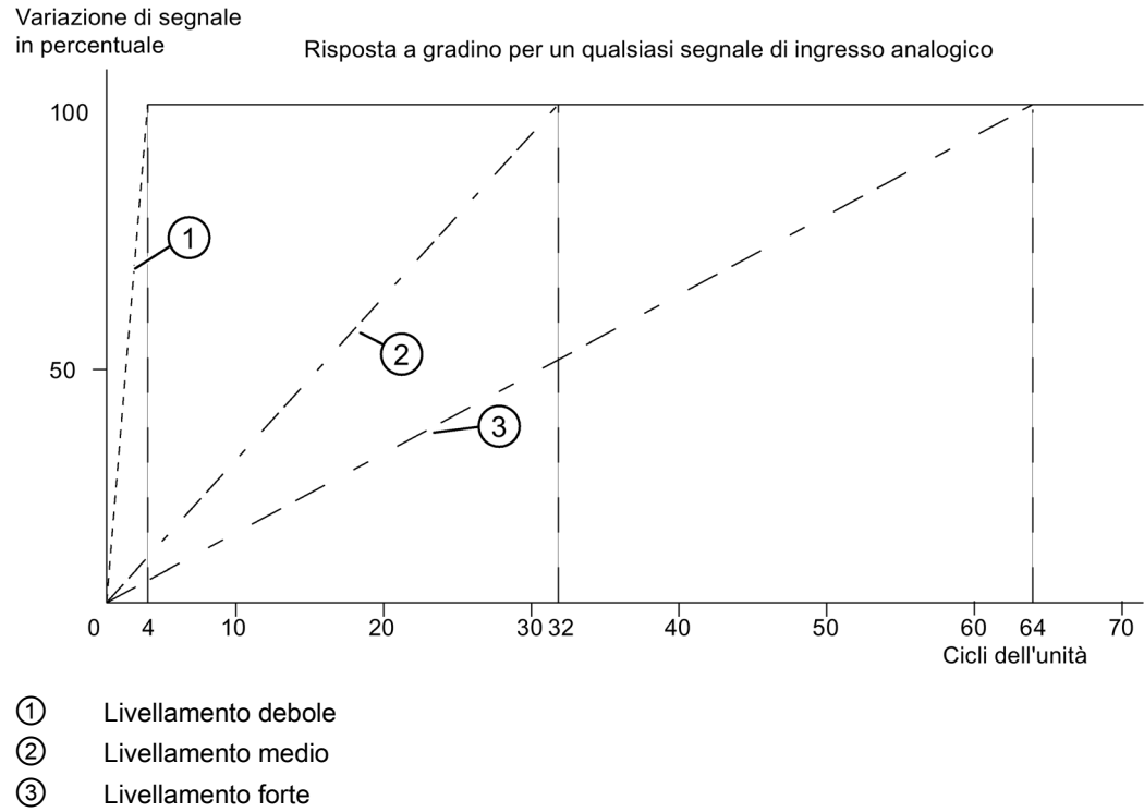
Figura 5-5 Esempio dell'influenza del livellamento sulla risposta a gradino del bit AI 8 x 14
