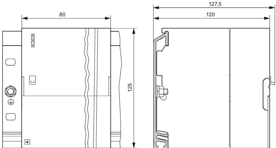
Figura C-14 Alimentatore PS 307; 10 A
