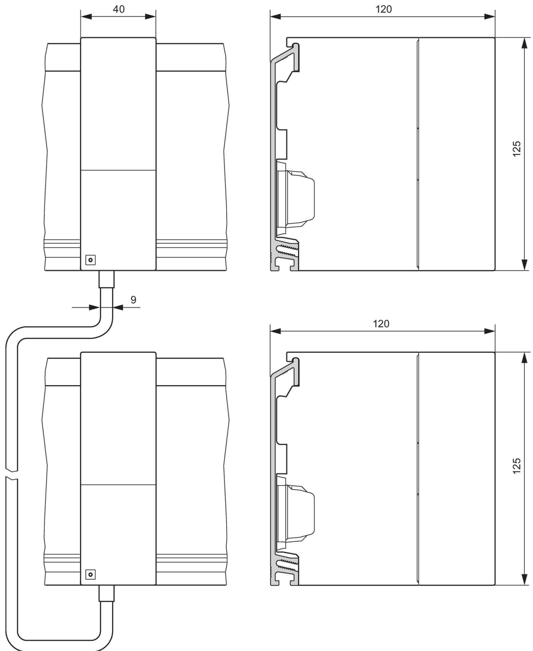
Figura C-17 Unità di interfaccia IM 365
